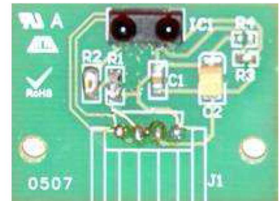
IRDA SENSE
